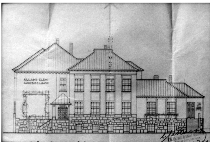
A zalaötvői iskola tervrajza 1929-ből
