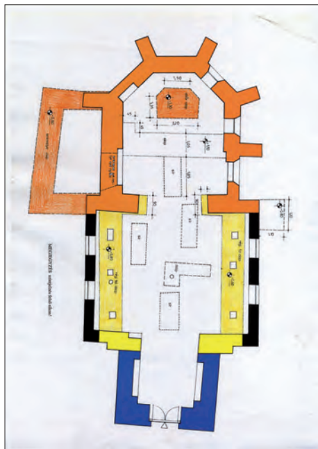
A nyírdzerzsi görögkatolikus templom periodizációs alaprajza. Barnássárga = 13. század; világos-sárga = 14. század eleje; barna = gótikus, 14–15. század fordulója; kék = barokk, 1797; fekete = újkori, 1927.
