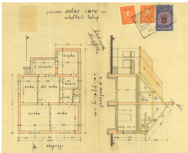
Botár Imre kertesházának terve (HU-MNL-JNSzML-V.473.c.-13393/1927)
