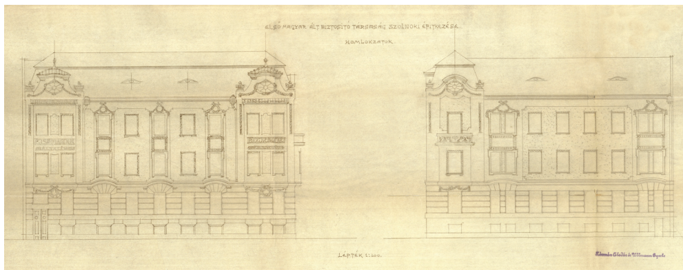
Első Magyar Biztosító Társaság szolnoki székháza (HU-MNL-JNSzML-V.473.c.-XIV 46/1905)
