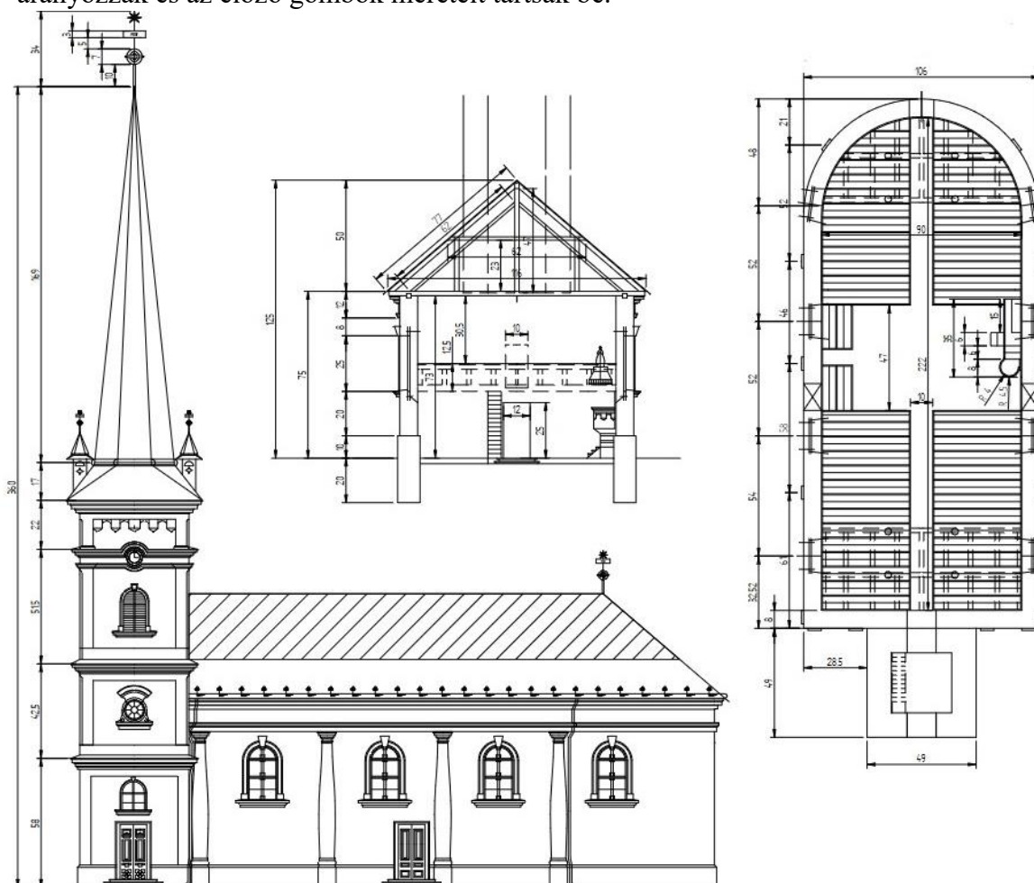
6. Rajzolta: Tétel Richárd Béla az eredeti tervek alapján
