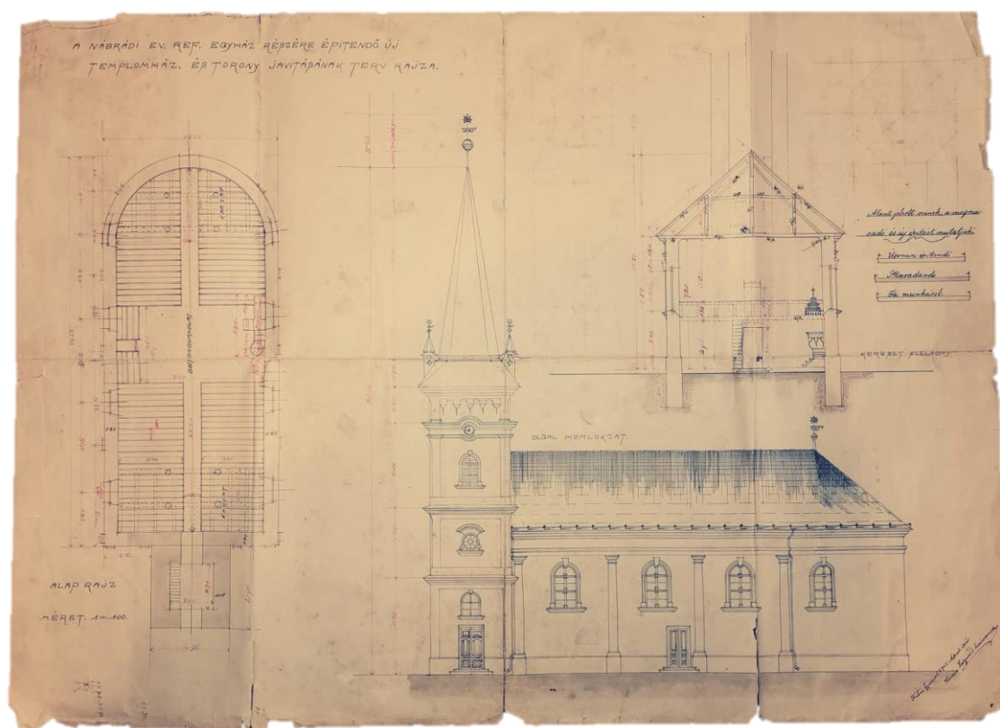
5. A nábrádi református templom eredeti tervrajza 1905
