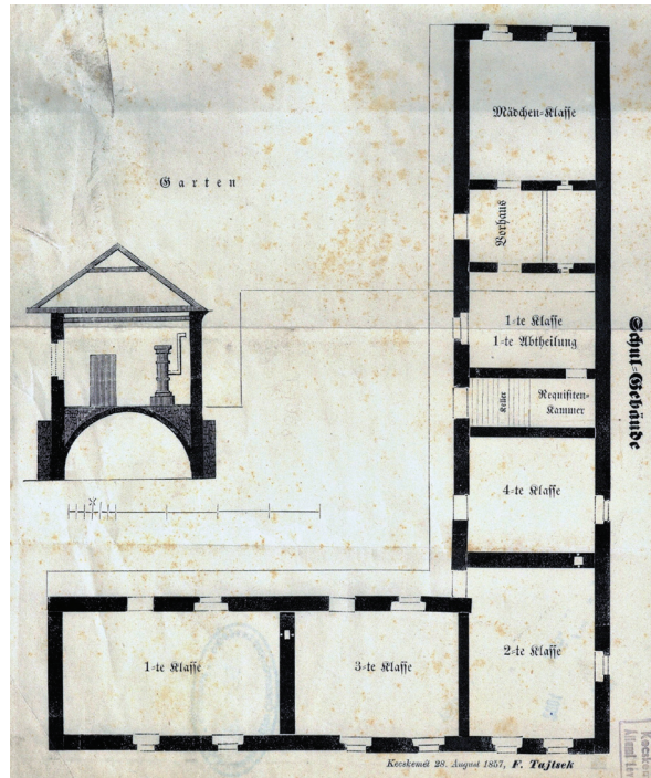
1. kép: Izraelita iskola tervrajza 1857-ből MNL BKML XV. 15.a.
