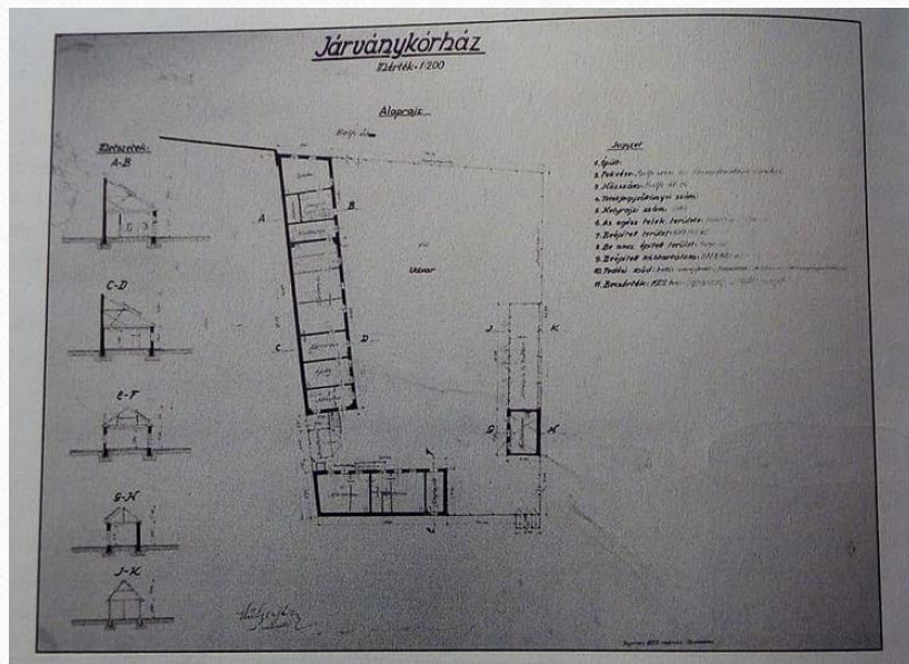
A Balfi utcai Járványkórház alaprajza, 1922. MNL GyMSM SL, SVLt
