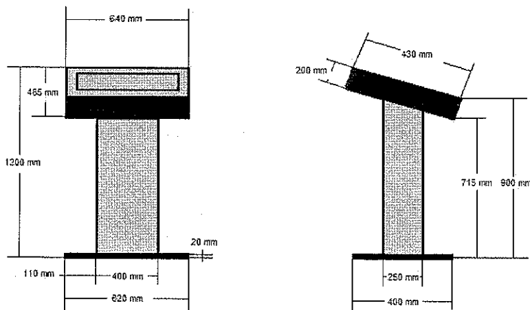
Debreceni Levéltár álló, döntött terminál méretezett vázlatrajza.
